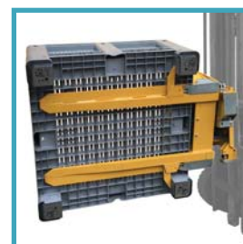
Sistema di bloccaggio Locking system
