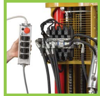
Distributore elettro-idraulico proporzionale Distribuidor electro hidráulico proporcional
