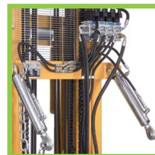
Kit doppio brandeggio Double tilting kit
